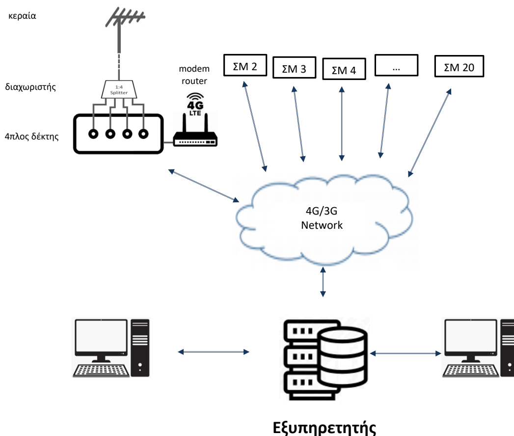
Σχήμα 1: Γενική αρχιτεκτονική συστήματος μέτρησης ποιότητας υπηρεσίας ψηφιακής τηλεοπτικής ευρυεκπομπής
