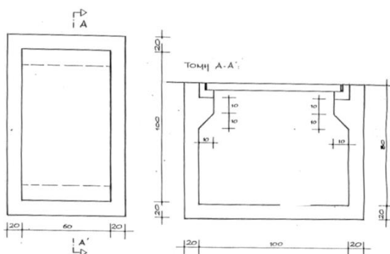
Εικόνα 10: Ενδεικτική κάτοψη και πλάγια όψη φρεατίου 60X80
