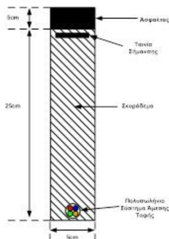
Εικόνα 8: Ενδεικτική τομή Μικροτάφρου επί διαμορφωμένης επιφάνειας
